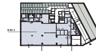
PŮDORYS PODLAŽÍ
